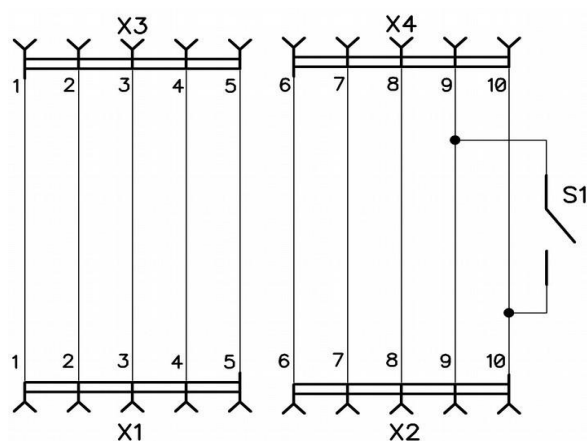
Рисунок А.2 – Схема принципиальная
