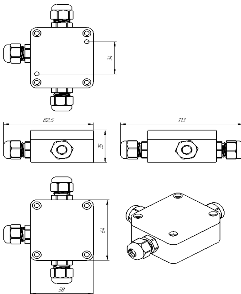
Рисунок А.1 – Габаритные и установочные размеры разветвителя интерфейса RS-422/485 ПР-3Д ТМП (исполнение 1)
