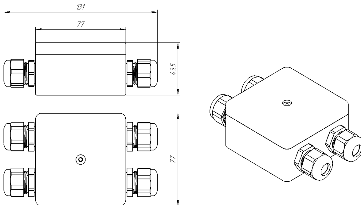
Рисунок А.1 – Габаритные и установочные размеры разветвителя интерфейса RS-422/485 ПР-4У (исполнение 2)
