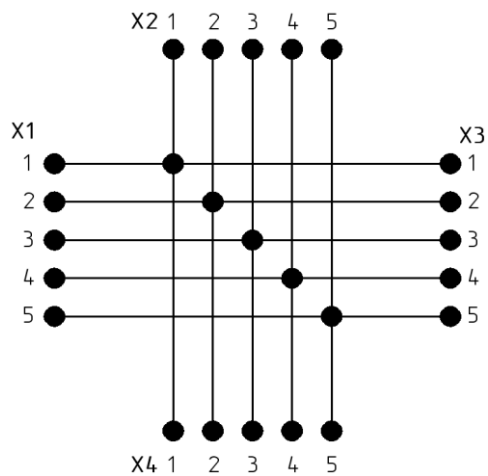
Рисунок А.2 – Схема принципиальная
