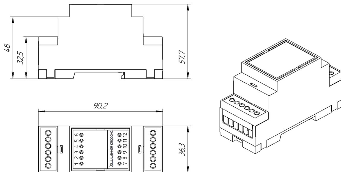
Рисунок А.1 – Установочные размеры УЗИП DIO-24-1-G
