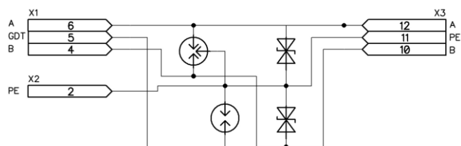
Рисунок А.2 – Схема УЗИП DIO-24-1-G
