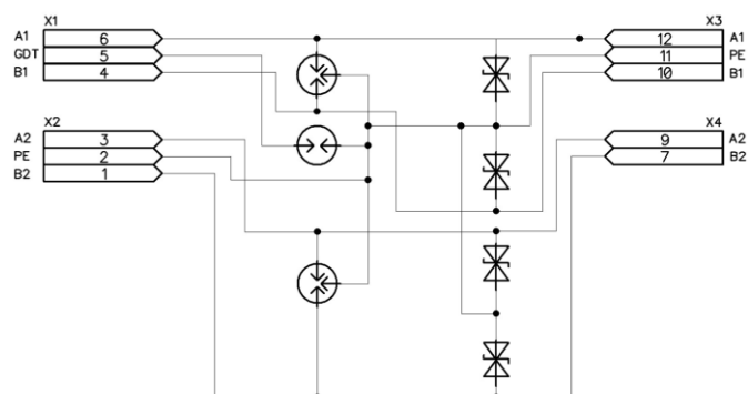
Рисунок А.2 – Схема УЗИП DIO-24-2-G
