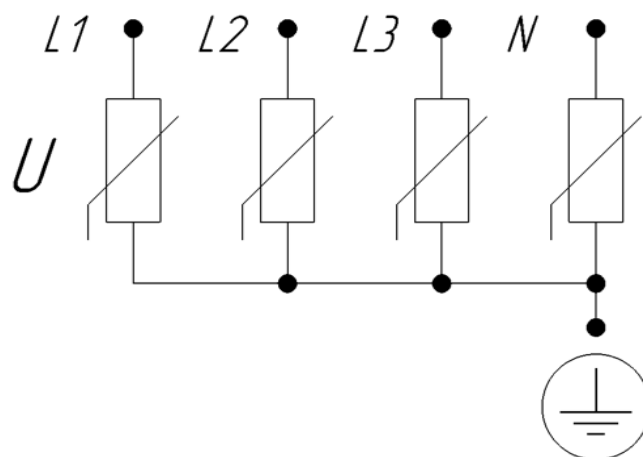
Рисунок Б.2 – Схема электрическая принципиальная
