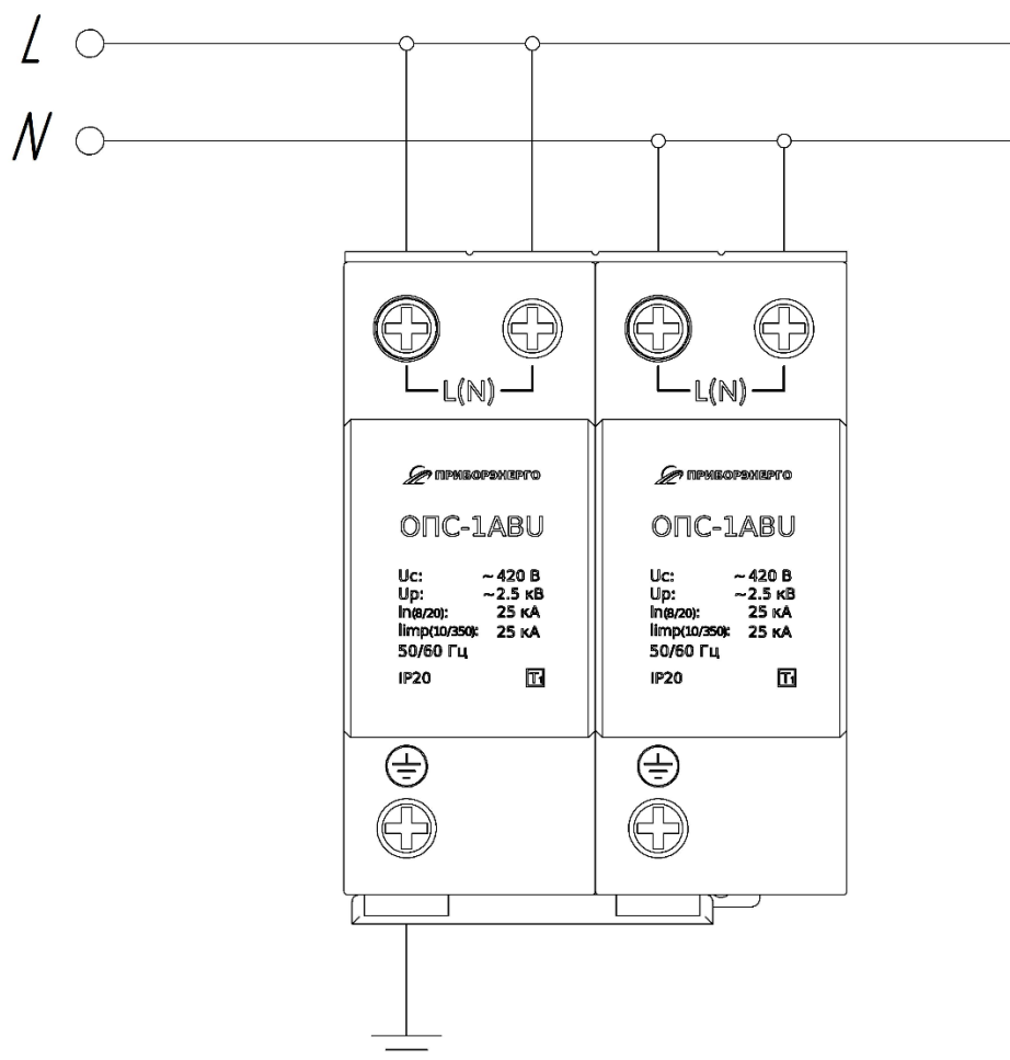
Рисунок Б.1 – Схема УЗИП ОПС-11В-2Р 1 класса
