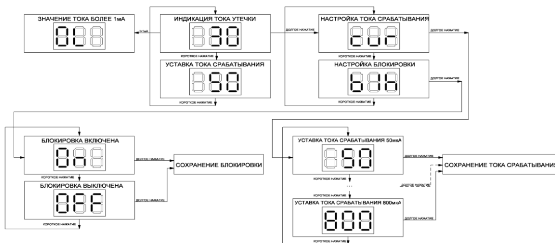
Рисунок 4 – Общая структура меню РКТУ-1М
