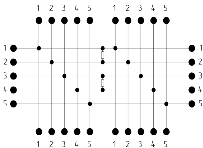
Рисунок А.2 – Схема принципиальная
