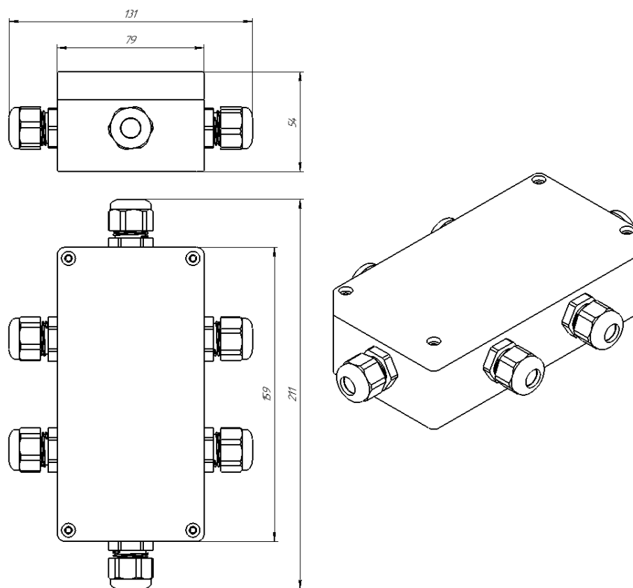
Рисунок А.1 – Габаритные и установочные размеры
