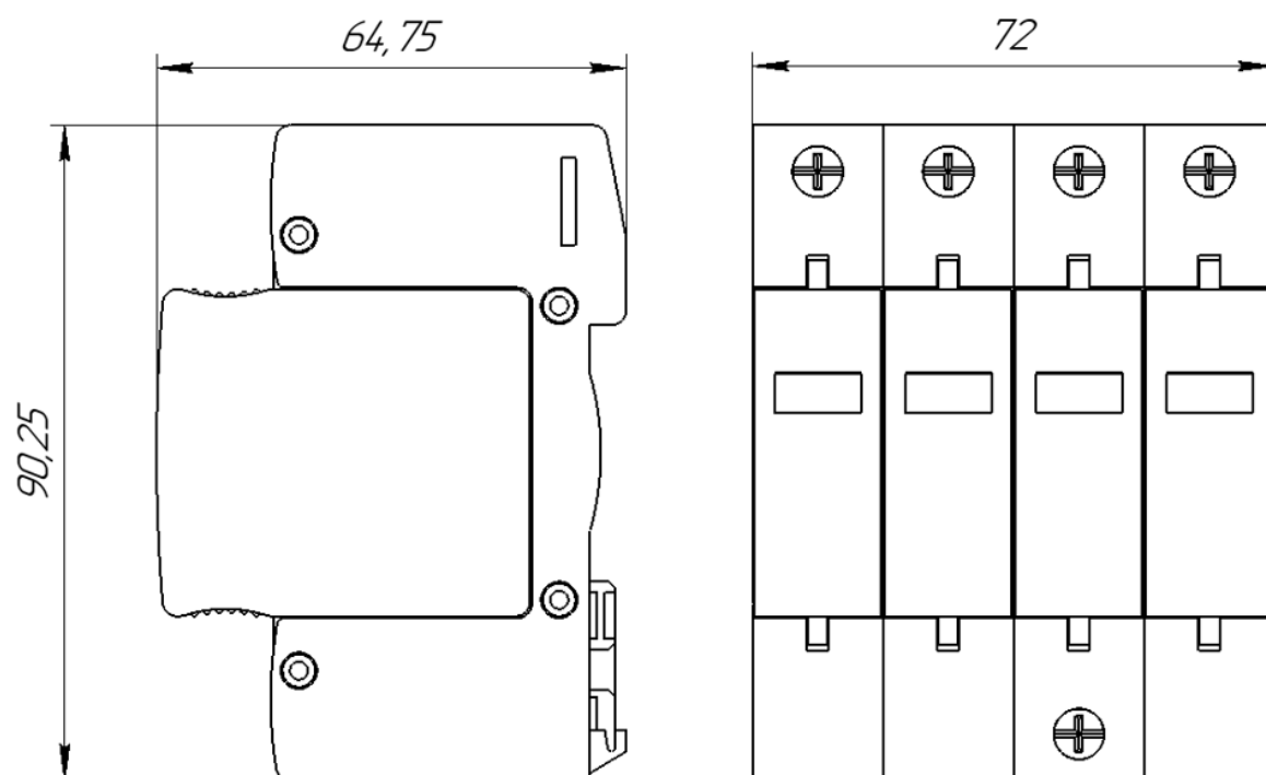
Рисунок А.1 – Габаритные размеры
