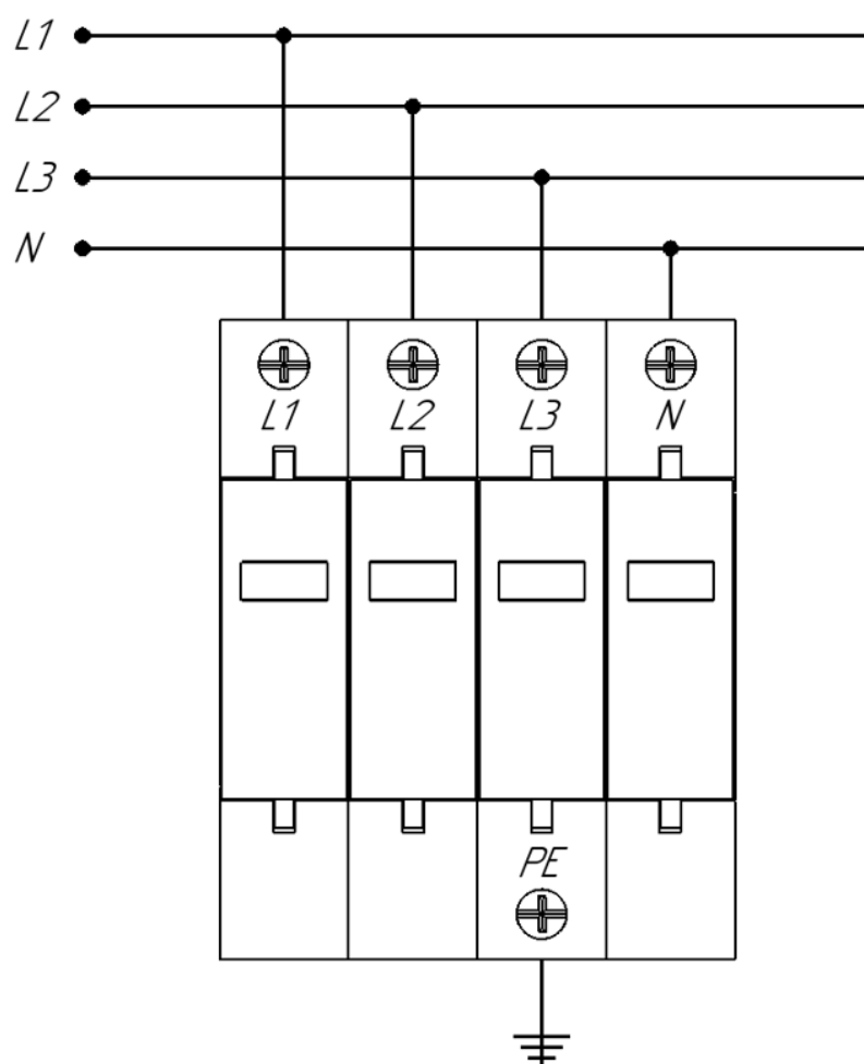
Рисунок Б.1 – Схема УЗИП ОПС-34Е-4РN 1+2 класса
