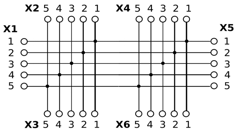
Рисунок А.2 – Схема принципиальная
