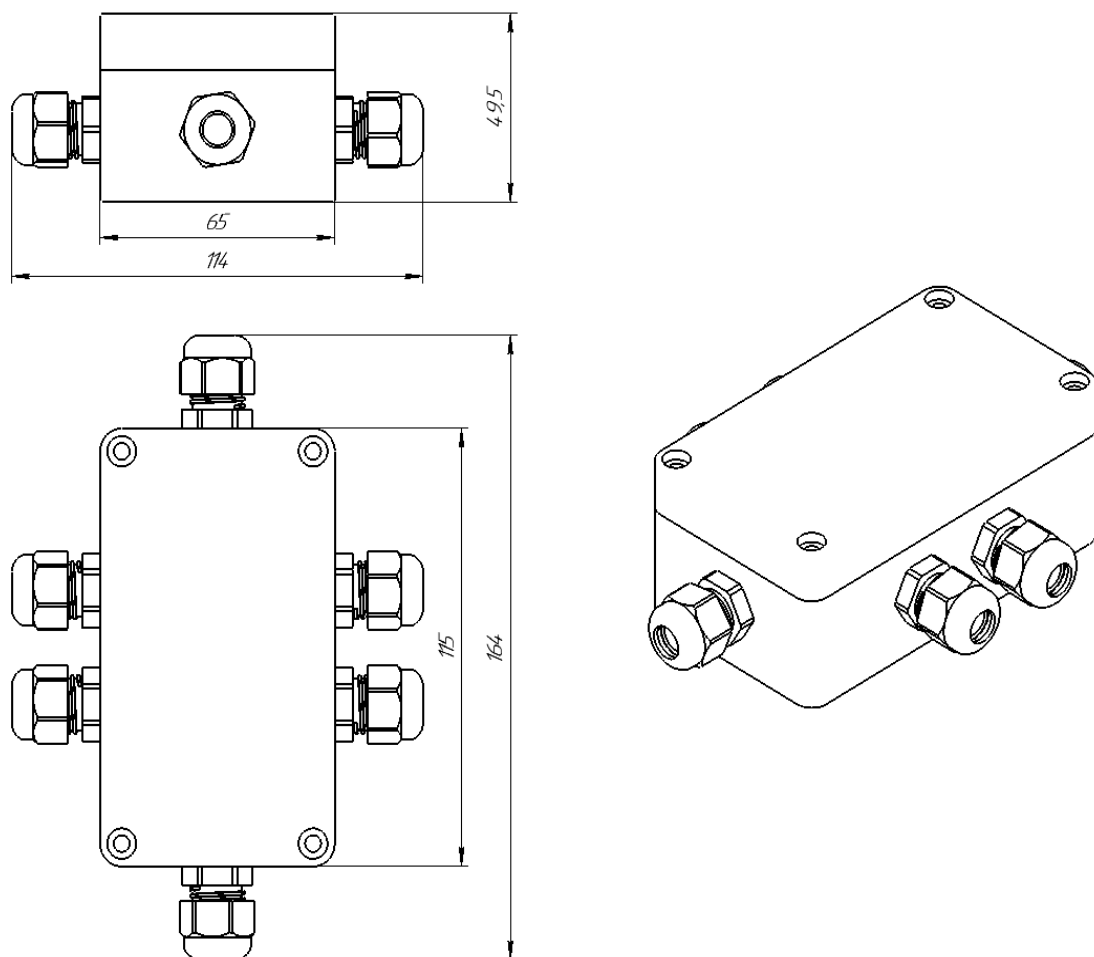
Рисунок А.1 – Габаритные и установочные размеры
