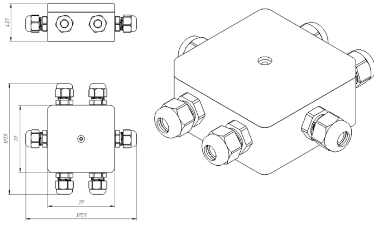
Рисунок А.1 – Габаритные и установочные размеры
