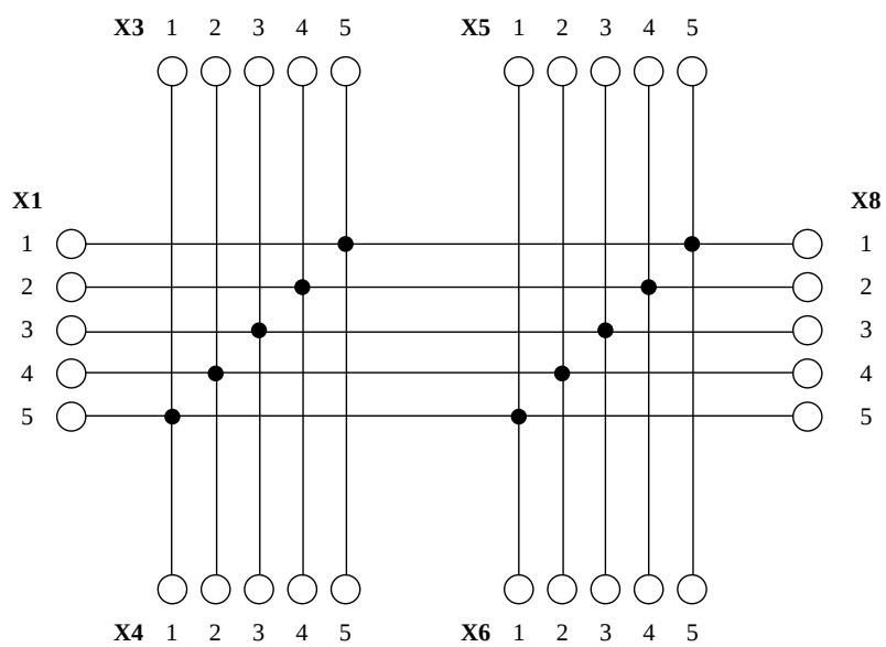
Рисунок А.2 – Схема принципиальная
