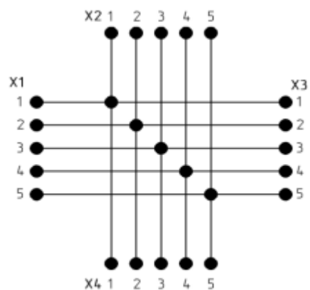
Рисунок А.2 – Схема принципиальная
