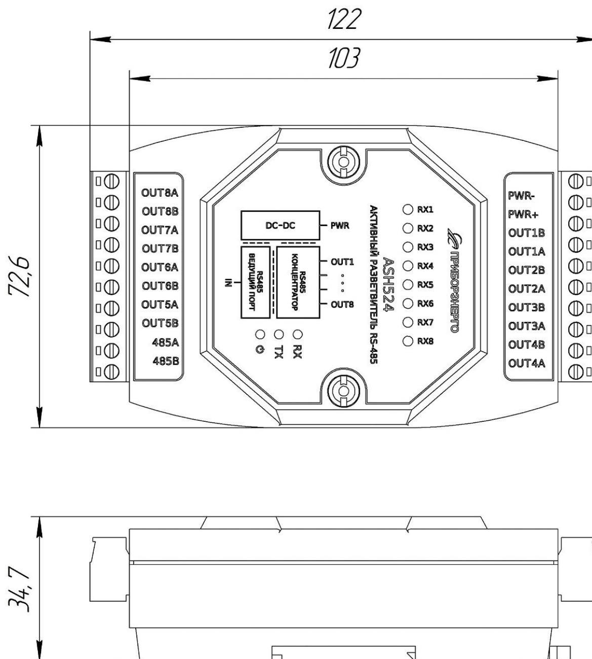
Рисунок А.1 – Габаритные размеры активного разветвителя интерфейса RS-485 ASH524
