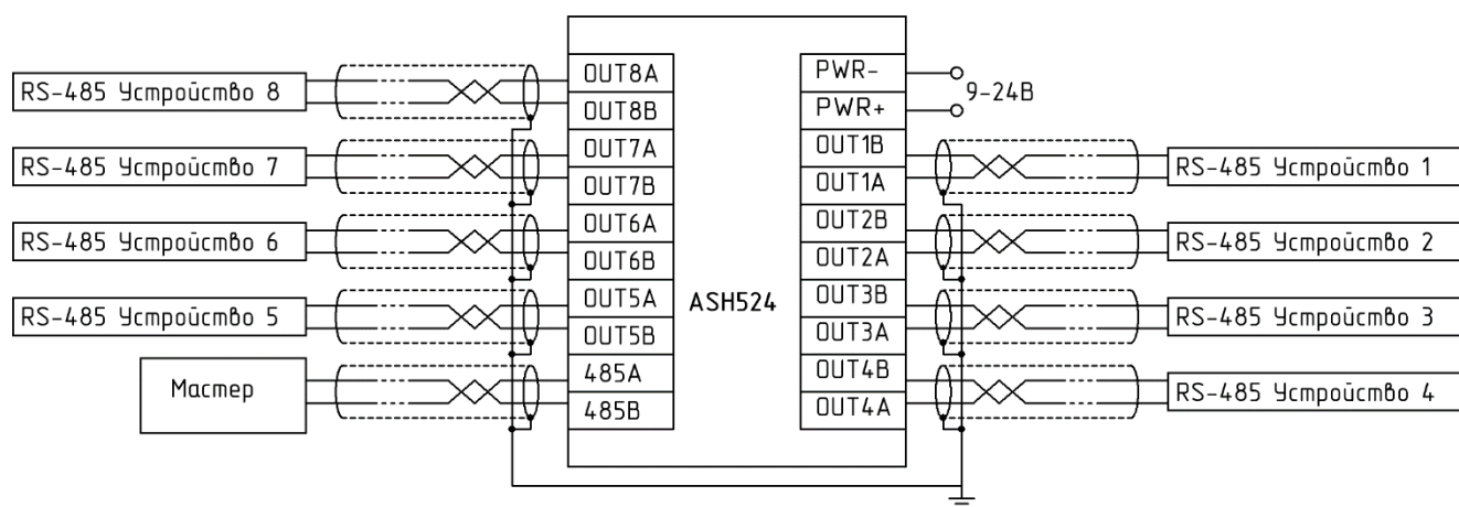
Рисунок А.2 – Схема подключения активного разветвителя интерфейса RS-485 ASH524
