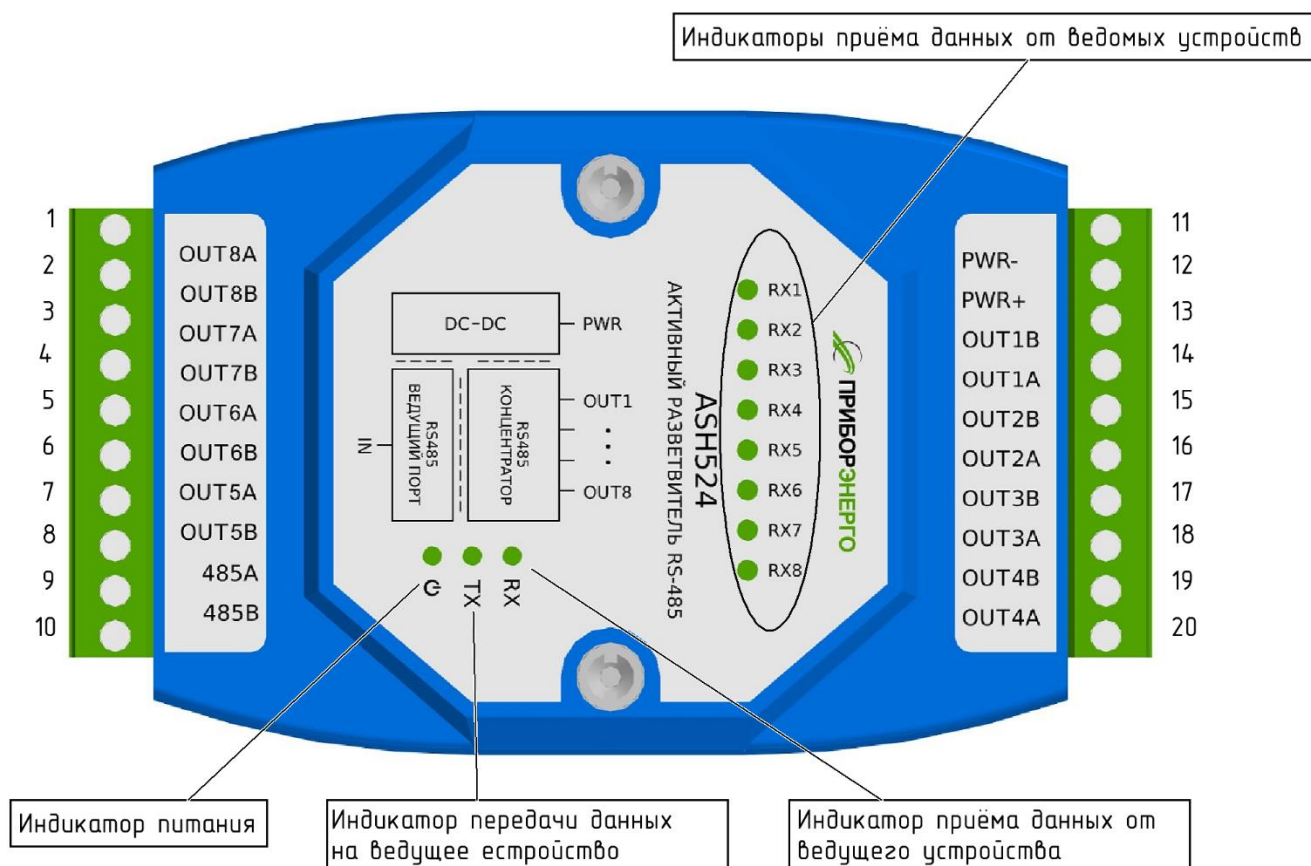
Рисунок А.3 – Схема расположения элементов управления, индикации и подключения активного разветвителя интерфейса RS-485 ASH524
