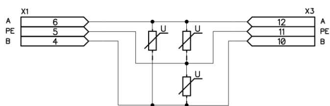
Рисунок А.2 – Схема УЗИП DIO-24-1-U
