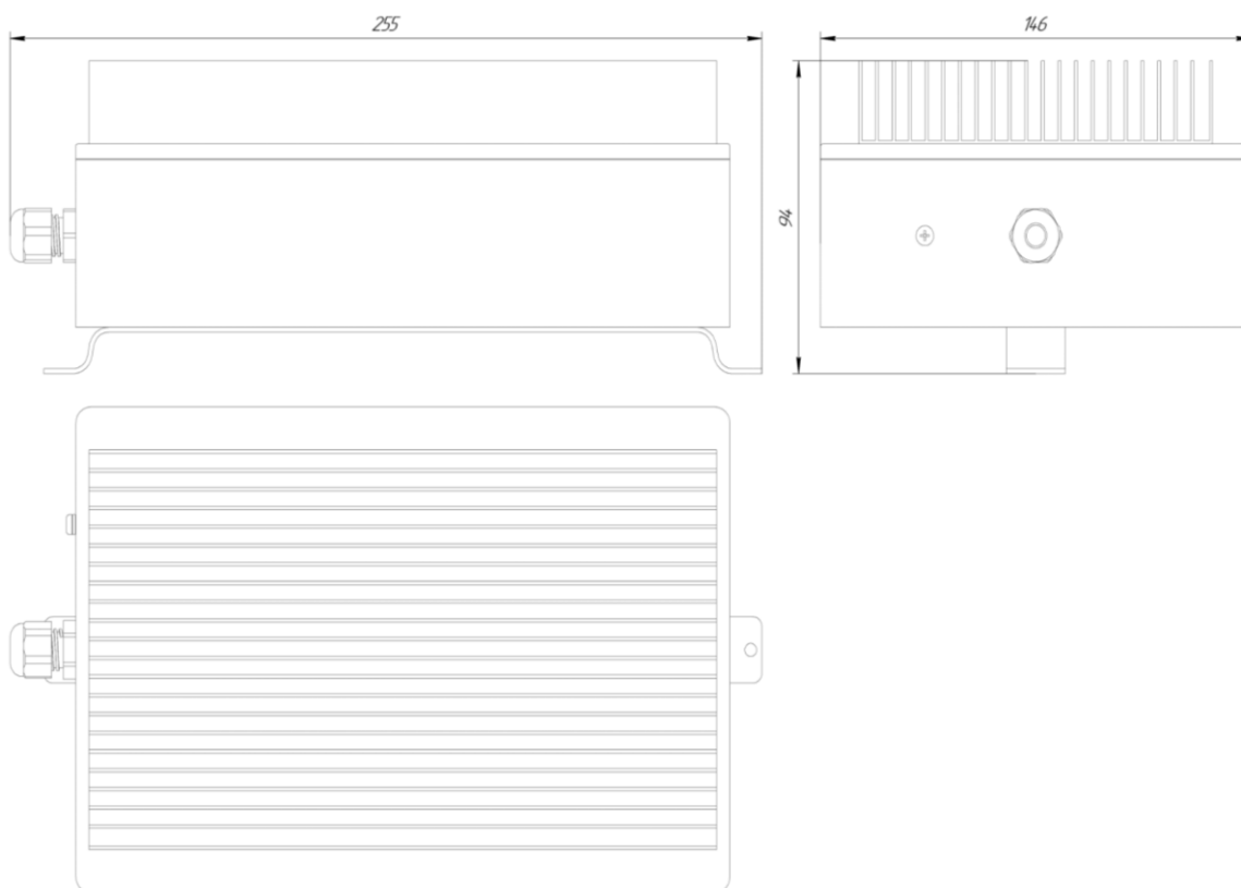
Рисунок А.2 – Габаритные размеры
