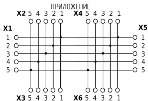
Рисунок А.2 – Схема принципиальная
