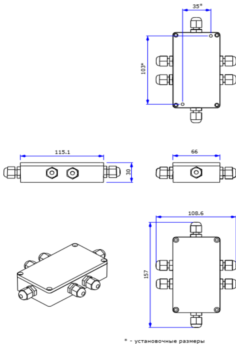
Рисунок А.1 – Габаритные и установочные размеры
