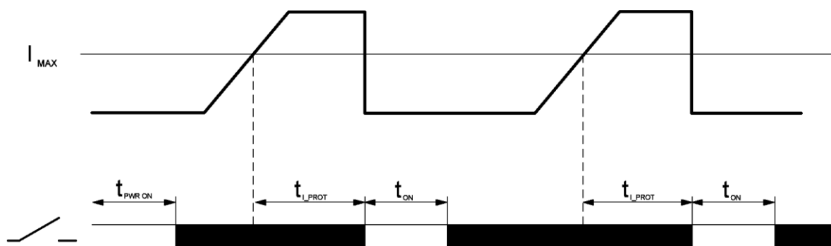
Рисунок 4 – Диаграмма работы реле контроля напряжения и тока VCR9310, срабатывание по току
