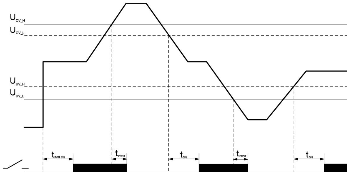
Рисунок 3 – Диаграмма работы реле контроля напряжения и тока VCR9310, срабатывание по напряжению
