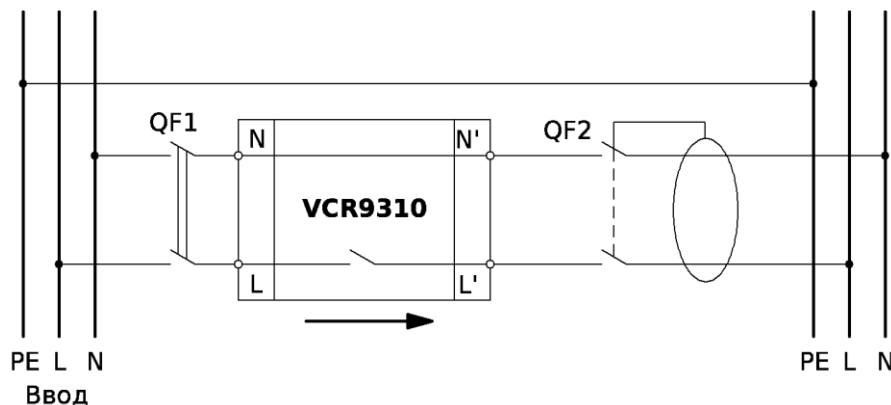
Рисунок 1 – Принципиальная схема подключения реле контроля напряжения и тока VCR9310
