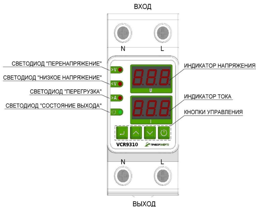
Рисунок 2 – Лицевая панель реле контроля напряжения и тока VCR9310
