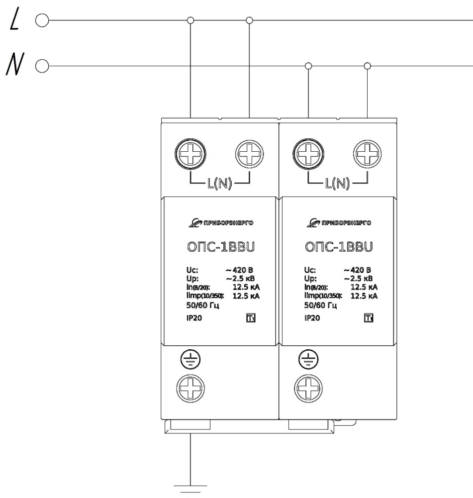
Рисунок Б.1 – Схема УЗИП ОПС-1ВВ-2РУ 1 класса
