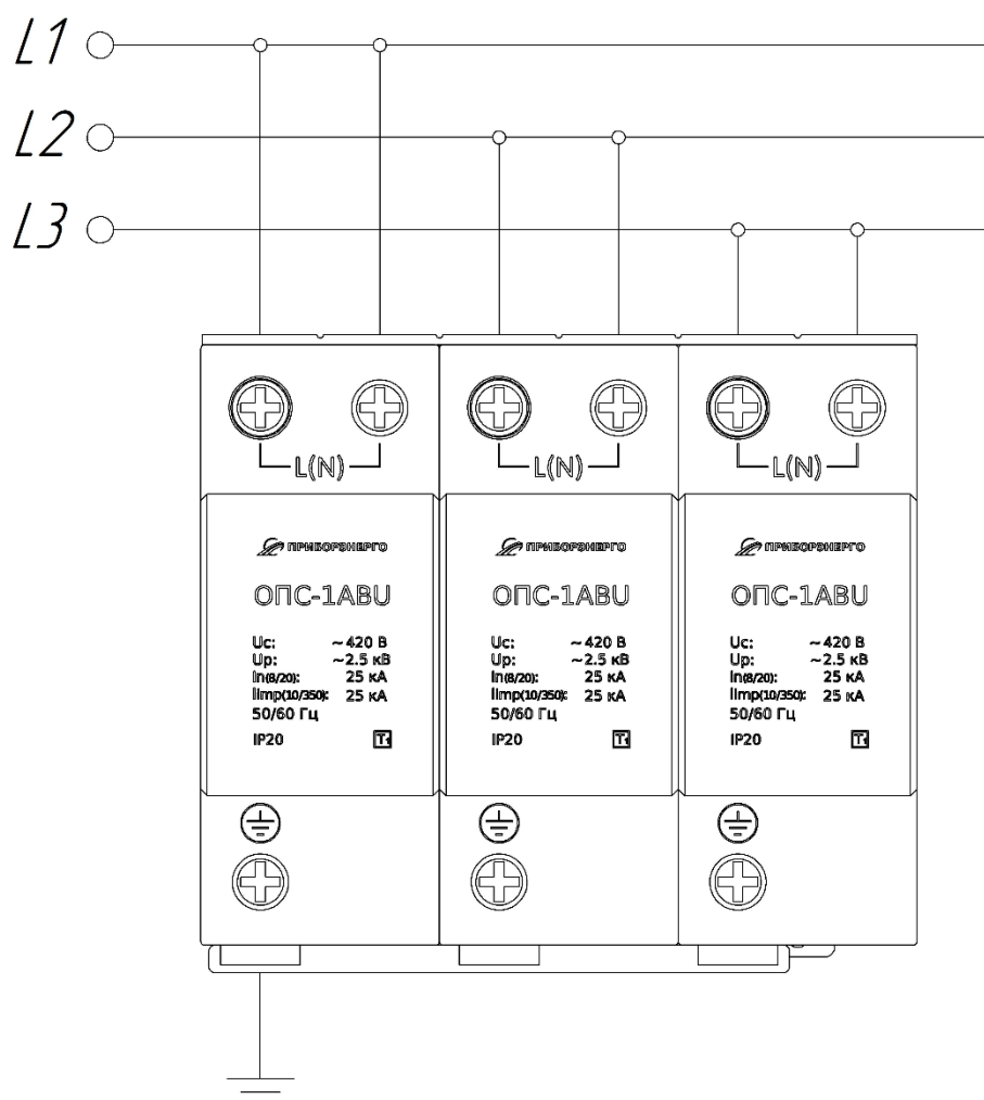
Рисунок Б.1 – Схема УЗИП ОПС-1АВ-3РУ 1 класса
