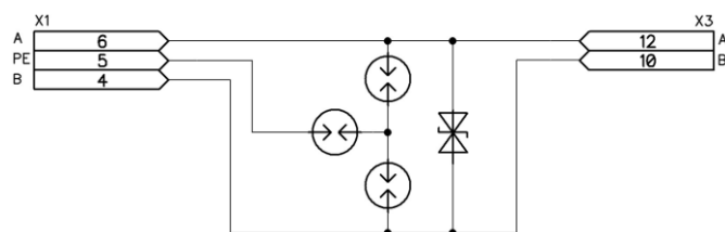
Рисунок А.2 – Схема УЗИП DIO-24-1-E
