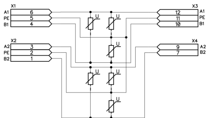
Рисунок А.2 – Схема УЗИП DIO-12-2-U
