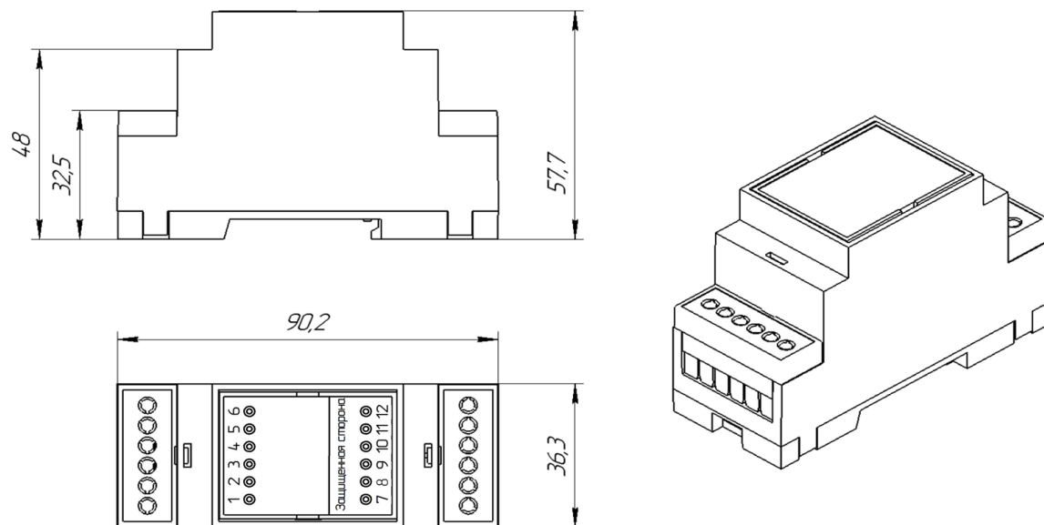
Рисунок А.1 – Установочные размеры УЗИП DIO-24-2-E
