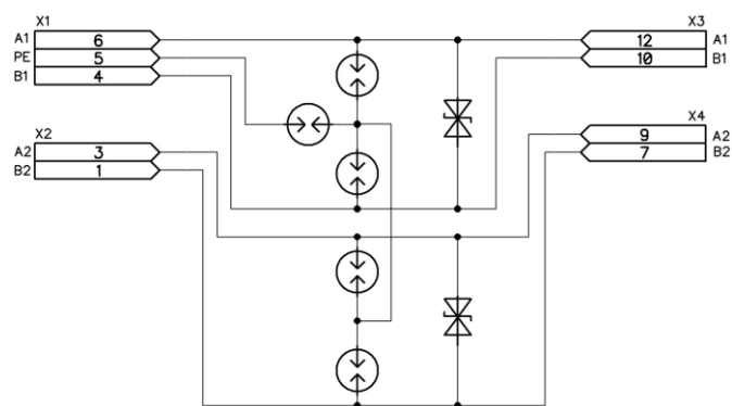
Рисунок А.2 – Схема УЗИП DIO-24-2-E
