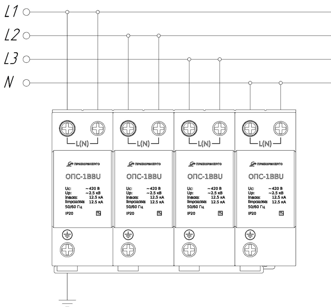
Рисунок Б.1 – Схема УЗИП ОПС-1ВВ-4РУ 1 класса
